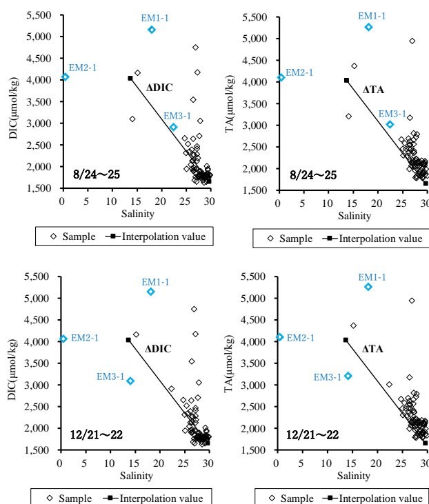
図-3.13 \Delta DIC, \Delta TA の算出結果【夏季, 冬季】、縦軸：DIC, 横軸：塩分, 白抜き黒点：採水サンプル, 黒点：境界地点, 白抜き水色点：河川側境界地点, 黒線：DIC と塩分の内挿値
