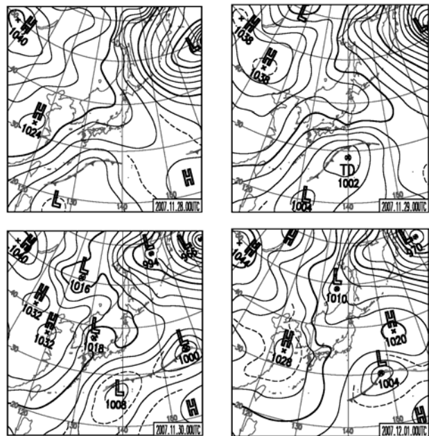
図-3.19 代表天気図（11月28日～12月1日）
