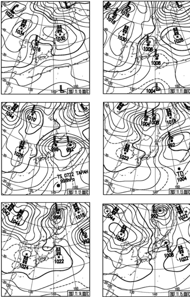
図-3.16 代表天気図（11月10日～11月15日）
