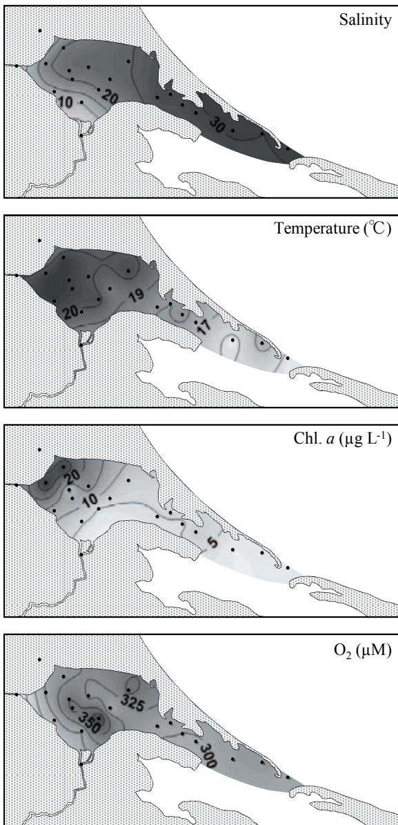
図-3 風蓮湖表層の塩分、水温、Chl. a 濃度、溶存酸素 ( O_2 ) 濃度の水平分布。
