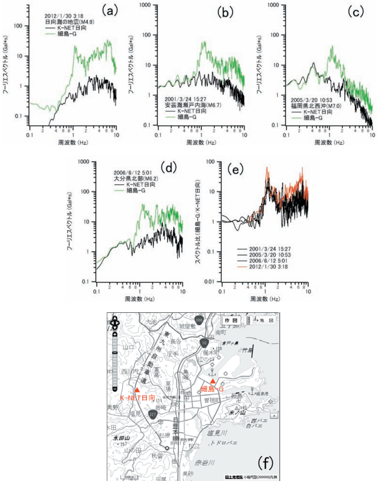
図-26 細島-GとK-NET日向で観測されたこれまでの主な記録のフーリエスペクトルとそれらの比 (下段は両地点の位置関係)
