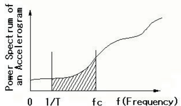
図-24 式(6)の意味するもの
