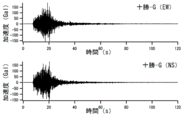
図-27 8月25日に十勝港で観測された加速度波形
