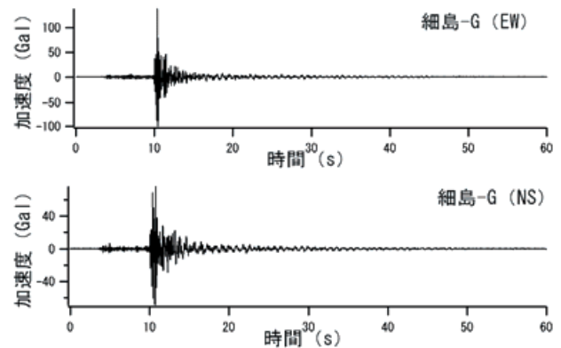
図-25 1 月 30 日に細島港で観測された加速度波形
