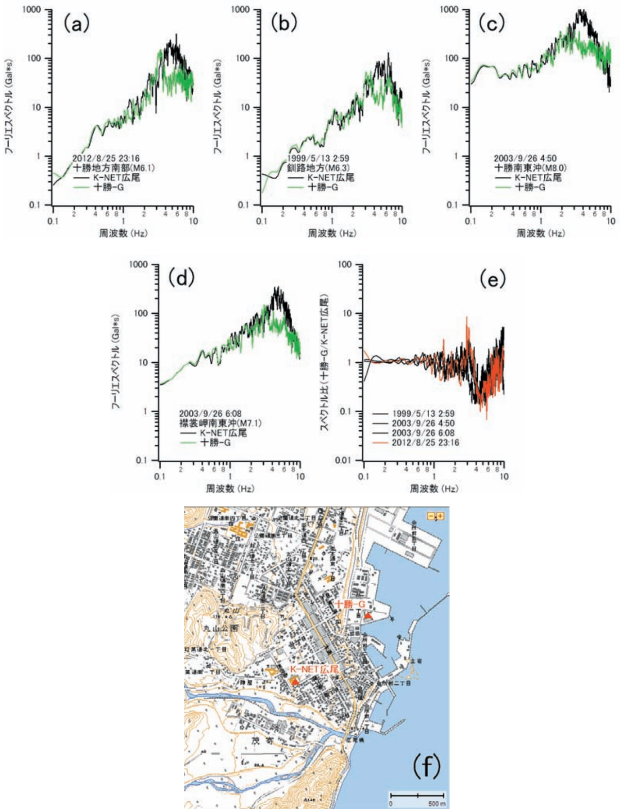
図-28 十勝-GとK-NET広尾で観測されたこれまでの主な記録のフーリエスペクトルとそれらの比 (下段は両地点の位置関係)
