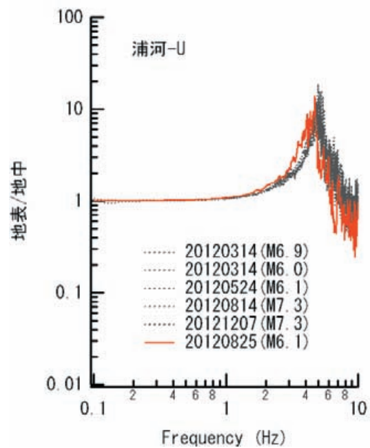
図-29 浦河港で観測された記録の地表と地中のスペクトル比。実線は8月25日の記録。破線は振幅の小さい記録。
