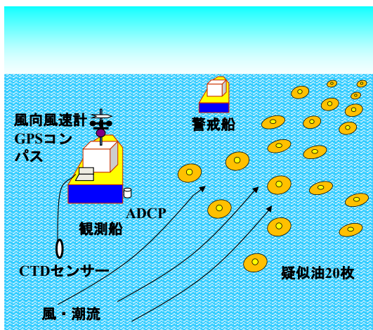
図- 4.7: 疑似油を用いた水平乱流拡散実験の模式図
