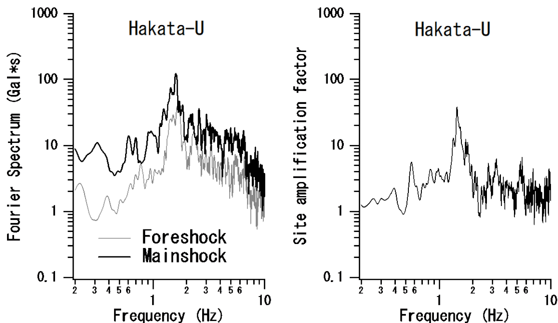
図-5.8 (左) 博多-Uで観測された前震・本震の加速度フーリエスペクトル. 縦軸: 加速度フーリエスペクトル, 横軸: 周波数. (右) 博多-Uのサイト増幅特性 ( http://www.ysk.nilim.go.jp/kakubu/kouwan/sisetu/sisetu.html ). 縦軸: サイト増幅特性, 横軸: 周波数.
