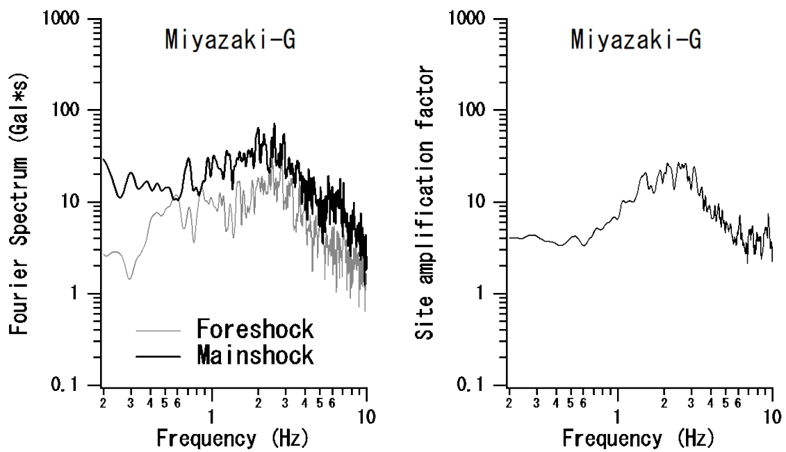
図-5.6 (左) 宮崎-G で観測された前震・本震の加速度フーリエスペクトル. 縦軸: 加速度フーリエスペクトル, 横軸: 周波数. (右) 宮崎-G のサイト増幅特性 3) . 縦軸: サイト増幅特性, 横軸: 周波数.
