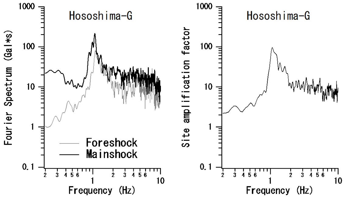
図-5.5 (左) 細島-G で観測された前震・本震の加速度フーリエスペクトル. 縦軸: 加速度フーリエスペクトル, 横軸: 周波数. (右) 細島-G のサイト増幅特性 3) . 縦軸: サイト増幅特性, 横軸: 周波数.
