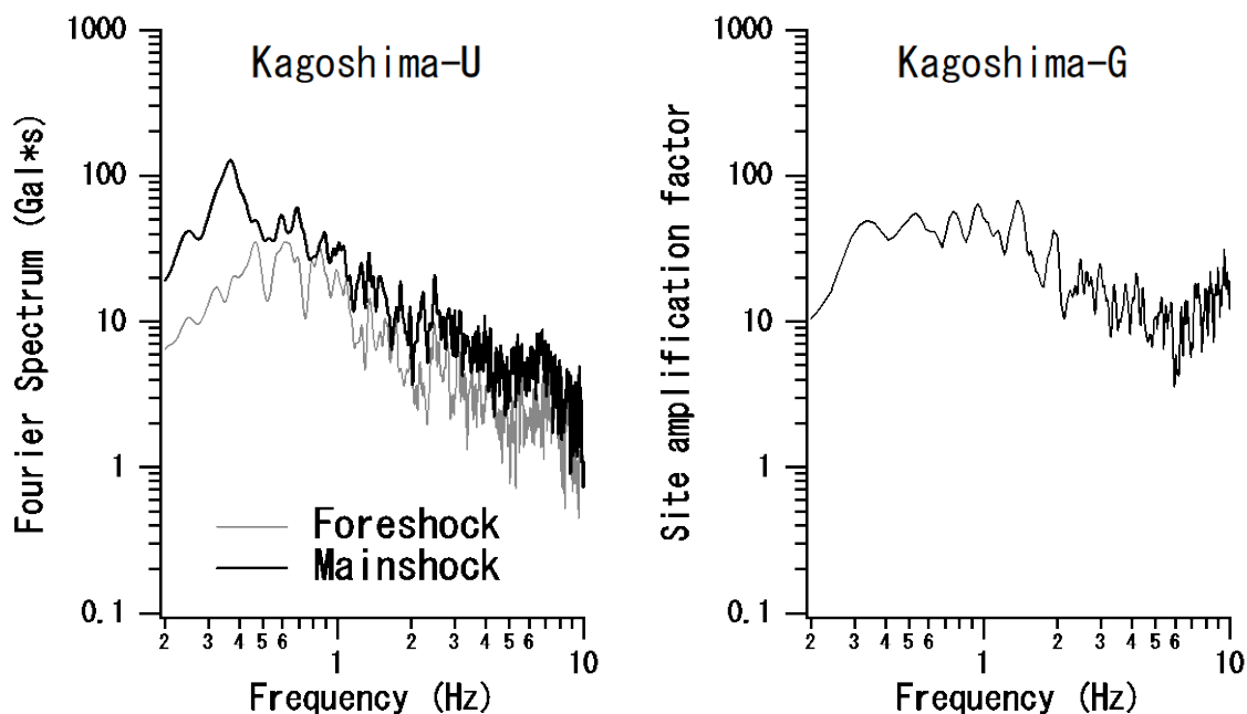
図-5.7 (左) 鹿児島-Uで観測された前震・本震の加速度フーリエスペクトル. 縦軸: 加速度フーリエスペクトル, 横軸: 周波数. (右) 鹿児島-G (=鹿児島-U) のサイト増幅特性 3) . 縦軸: サイト増幅特性, 横軸: 周波数.
