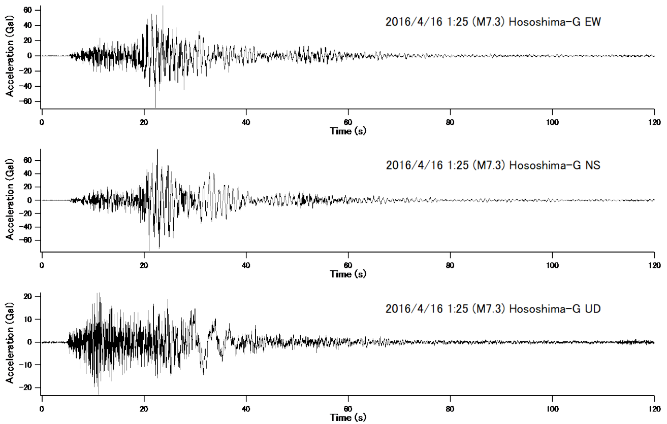
図-5.4 細島-G で観測された本震の3成分の加速度波形. 縦軸: 加速度, 横軸: 時間.
