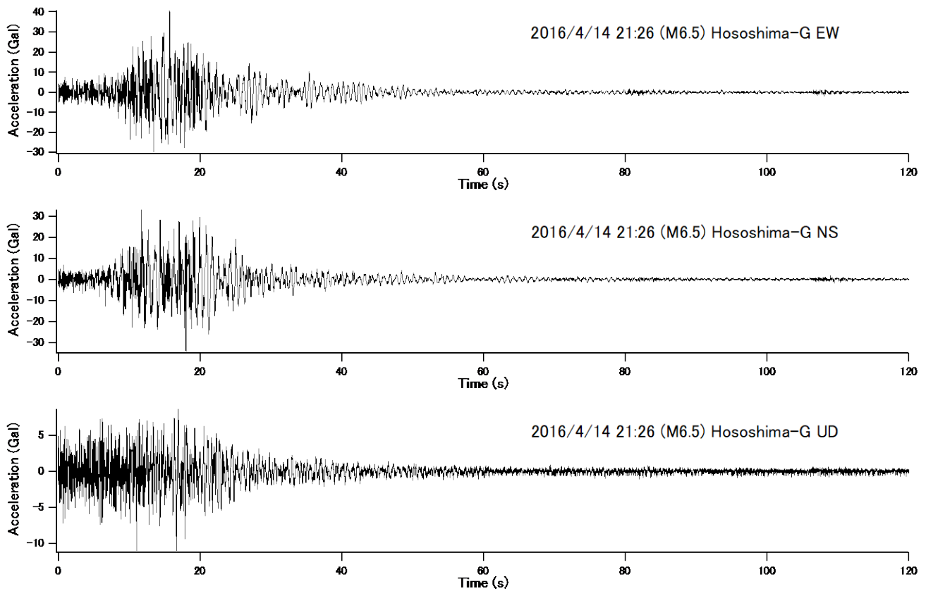
図-5.3 細島-G で観測された前震の3成分の加速度波形. 縦軸: 加速度, 横軸: 時間.
