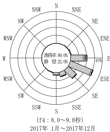
付図-B.3.78 宮崎日向沖 波高・波向別出現頻度図(連続観測, f2, f3, f4, f5, 全周期帯)
