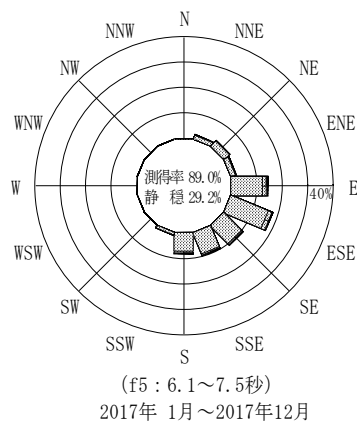
付図-B.3.78 宮崎日向沖 波高・波向別出現頻度図(連続観測, f2, f3, f4, f5, 全周期帯)
