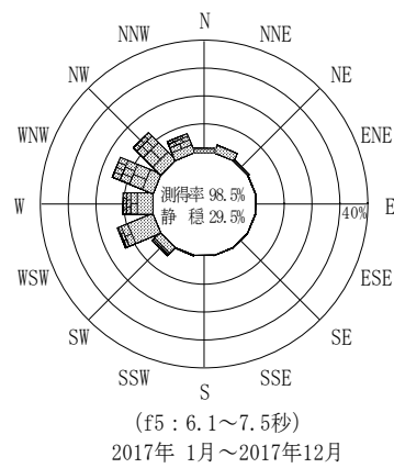
付図-B.3.61 青森西岸沖 波高・波向別出現頻度図(連続観測, f2, f3, f4, f5, 全周期帯)
