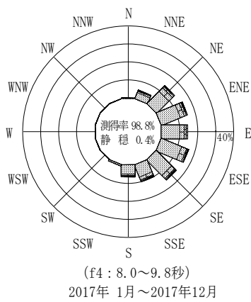
付図-B.3.70 福島県沖 波高・波向別出現頻度図(連続観測, f2, f3, f4, f5, 全周期帯)
