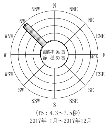
付図-B. 3. 60 石垣沖 波高・波向別出現頻度図(連続観測, f2, f3, f4, f5, 全周期帯)
