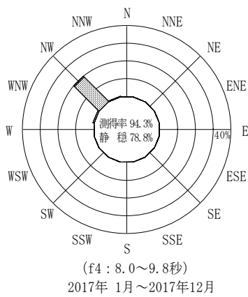
付図-B. 3. 60 石垣沖 波高・波向別出現頻度図(連続観測, f2, f3, f4, f5, 全周期帯)
