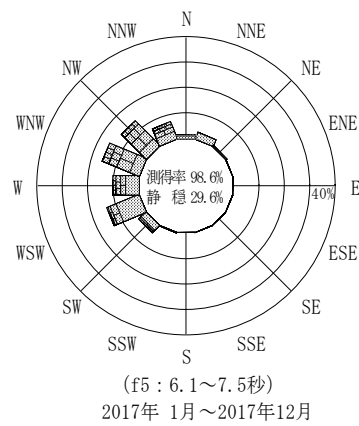
付図-A.3.61 青森西岸沖 波高・波向別出現頻度図 (f2, f3, f4, f5, 全周期帯)
