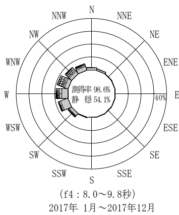
付図-A.3.61 青森西岸沖 波高・波向別出現頻度図 (f2, f3, f4, f5, 全周期帯)
