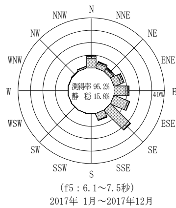
付図-A.3.64 青森東岸沖 波高・波向別出現頻度図 (f2, f3, f4, f5, 全周期帯)
