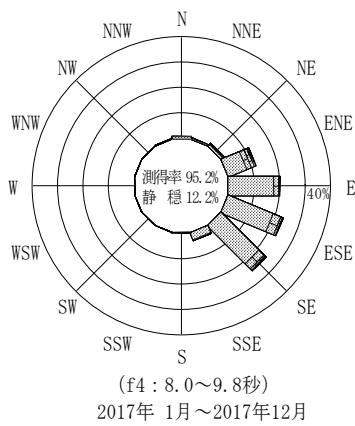
付図-A.3.64 青森東岸沖 波高・波向別出現頻度図 (f2, f3, f4, f5, 全周期帯)
