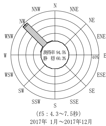
付図-A.3.60 石垣沖 波高・波向別出現頻度図 (f2, f3, f4, f5, 全周期帯)
