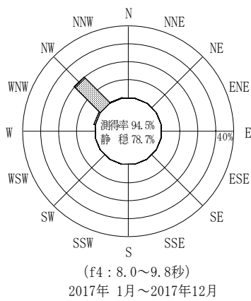
付図-A.3.60 石垣沖 波高・波向別出現頻度図 (f2, f3, f4, f5, 全周期帯)
