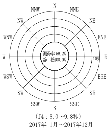
付図-A.3.54 苅田 波高・波向別出現頻度図 (f2, f3, f4, f5, 全周期帯)
