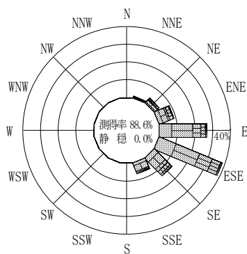
付図－B. 2. 40 常陸那珂 波高・波向別出現頻度図（連続観測）
