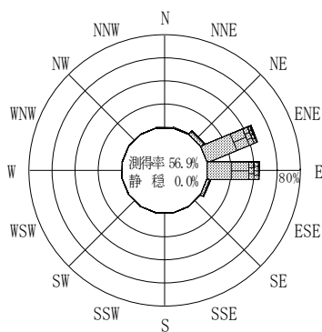
付図－B. 2. 35 釜石 波高・波向別出現頻度図（連続観測）
