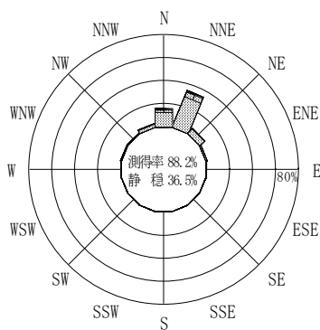
付図－B. 2. 10 富山 波高・波向別出現頻度図（連続観測）
