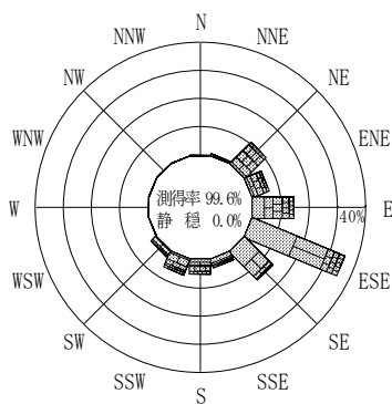
付図－A.2.76 高知室戸岬沖 波高・波向別出現頻度図
