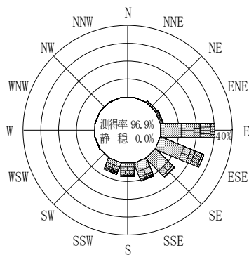
付図－A. 2. 73 三重尾鷲沖 波高・波向別出現頻度図
