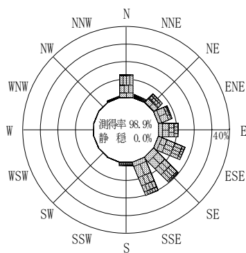
付図－A. 2. 65 岩手北部沖 波高・波向別出現頻度図
