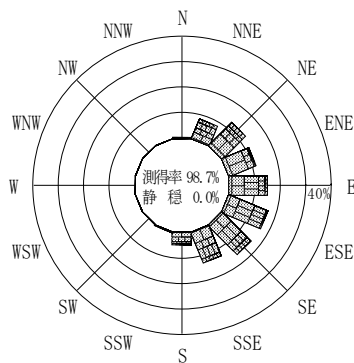
付図－A. 2. 70 福島県沖 波高・波向別出現頻度図
