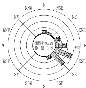
付図－A. 2. 64 青森東岸沖 波高・波向別出現頻度図
