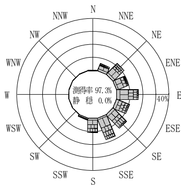
付図－A. 2. 68 宮城北部沖 波高・波向別出現頻度図
