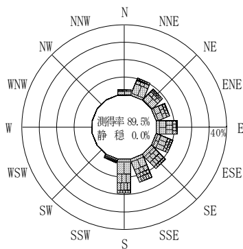
付図－A. 2. 67 岩手南部沖 波高・波向別出現頻度図
