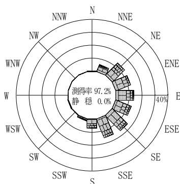
付図－A. 2. 69 宮城中部沖 波高・波向別出現頻度図
