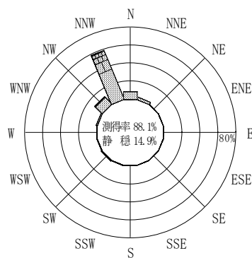
付図－A. 2. 59 平良沖 波高・波向別出現頻度図
