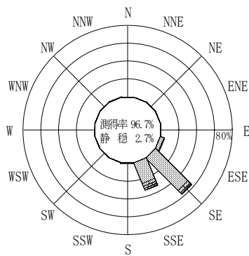
付図－A. 2. 56 志布志湾 波高・波向別出現頻度図
