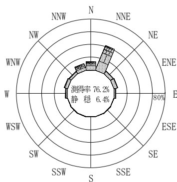
付図-A.2.22 玄界灘 波高・波向別出現頻度図
