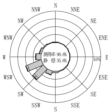
付図-A.2.23 伊王島 波高・波向別出現頻度図
