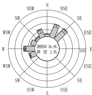
付図-A.2.25 名瀬 波高・波向別出現頻度図
