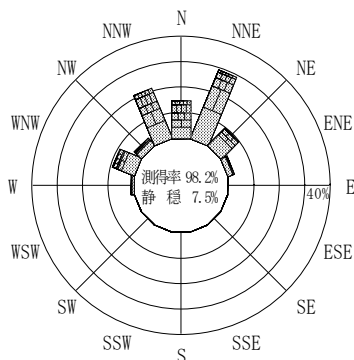
付図－A.2.18 鳥取 波高・波向別出現頻度図
