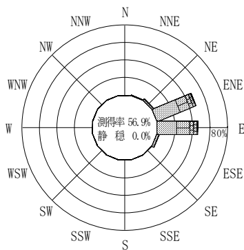
付図－A. 2. 35 釜石 波高・波向別出現頻度図
