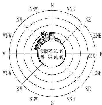
付図－A.2.14 福井 波高・波向別出現頻度図
