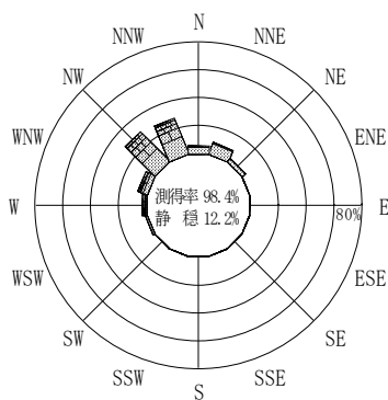
付図－A.2.9 直江津 波高・波向別出現頻度図
