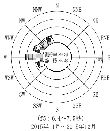
付図-B.3.1 留萌 波高・波向別出現頻度図 (連続観測, f2, f3, f4, f5, 全周期帯)
