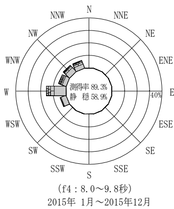
付図-B.3.1 留萌 波高・波向別出現頻度図 (連続観測, f2, f3, f4, f5, 全周期帯)
