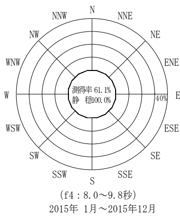
付図-B.3.54 苅田 波高・波向別出現頻度図 (連続観測, f2, f3, f4, f5, 全周期帯)
