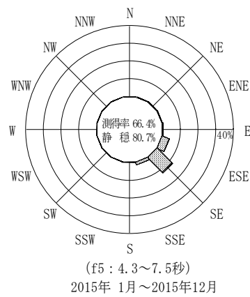
付図-B.3.50 小松島 波高・波向別出現頻度図(連続観測, f2, f3, f4, f5, 全周期帯)
