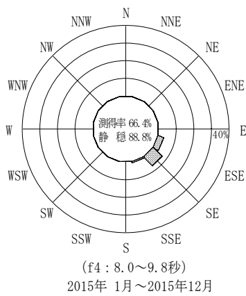
付図-B.3.50 小松島 波高・波向別出現頻度図(連続観測, f2, f3, f4, f5, 全周期帯)
