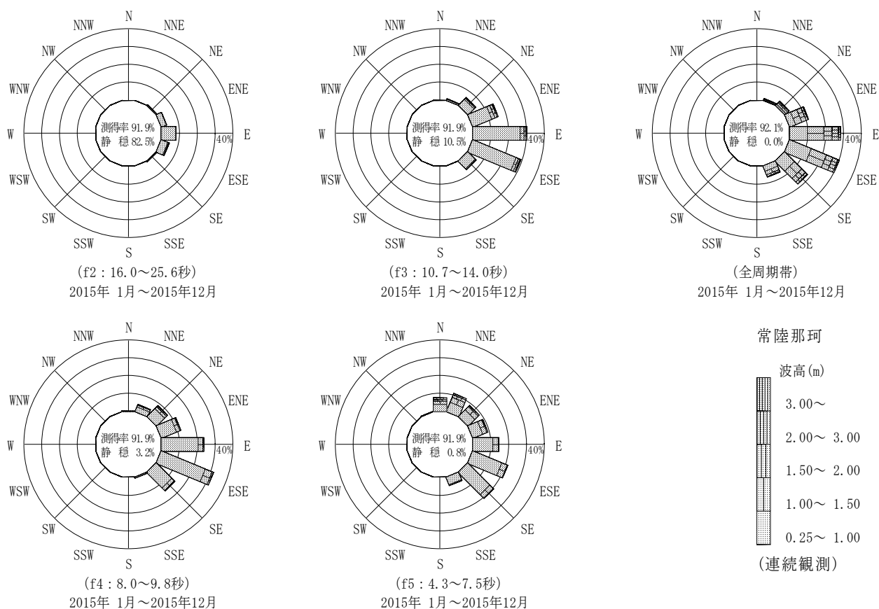
付図-B.3.40 常陸那珂 波高・波向別出現頻度図 (連続観測, f2, f3, f4, f5, 全周期帯)
