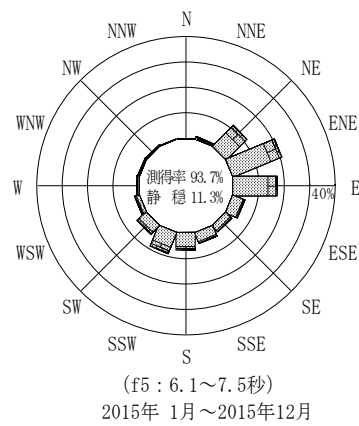
付図-A.3.76 高知室戸岬沖 波高・波向別出現頻度図 (f2, f3, f4, f5, 全周期帯)
