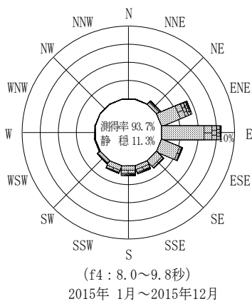
付図-A.3.76 高知室戸岬沖 波高・波向別出現頻度図 (f2, f3, f4, f5, 全周期帯)
