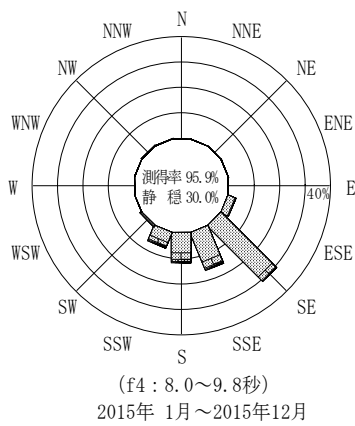
付図-A.3.74 和歌山南西沖 波高・波向別出現頻度図 (f2, f3, f4, f5, 全周期帯)
