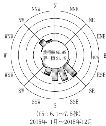
付図-A.3.74 和歌山南西沖 波高・波向別出現頻度図 (f2, f3, f4, f5, 全周期帯)
