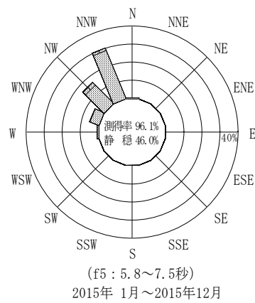
付図-A.3.59 平良沖 波高・波向別出現頻度図 (f2, f3, f4, f5, 全周期帯)
