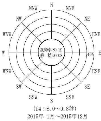
付図-A.3.57 鹿児島 波高・波向別出現頻度図 (f2, f3, f4, f5, 全周期帯)
