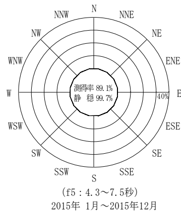
付図-A.3.57 鹿児島 波高・波向別出現頻度図 (f2, f3, f4, f5, 全周期帯)
