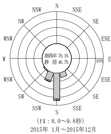
付図-A.3.51 室津 波高・波向別出現頻度図 (f2, f3, f4, f5, 全周期帯)
