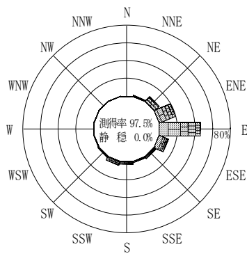
付図－B.2.76 高知室戸岬沖 波高・波向別出現頻度図（連続観測）
