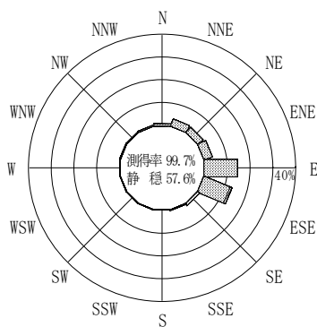
付図－B. 2. 54 荇田 波高・波向別出現頻度図（連続観測）
