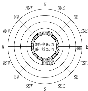
付図－B.2.42 第二海堡 波高・波向別出現頻度図（連続観測）
