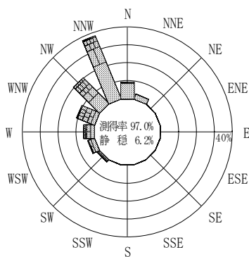
付図－B.2.13 金沢 波高・波向別出現頻度図（連続観測）
