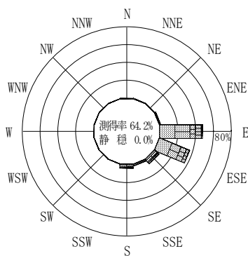
付図－A. 2. 78 宮崎日向沖 波高・波向別出現頻度図
