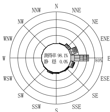
付図－A.2.76 高知室戸岬沖 波高・波向別出現頻度図
