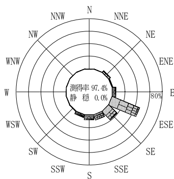
付図－A. 2. 75 徳島海陽沖 波高・波向別出現頻度図
